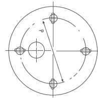
外形尺寸图
